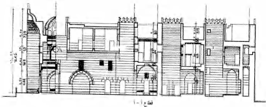
شكل رقم (٦): مدرسة الظاهر برقوق بالحناسين - مسقط أفقي وقطاع رأسي.
